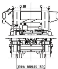
(前後輪) 1850
