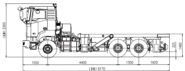
(全長) 9170
