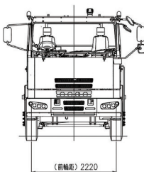
(前後輪) 2220
