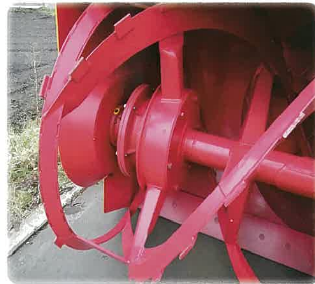
●オーガ油圧クラッチ式シャーピンレス装置仕様 (運転室内操作復帰型)
